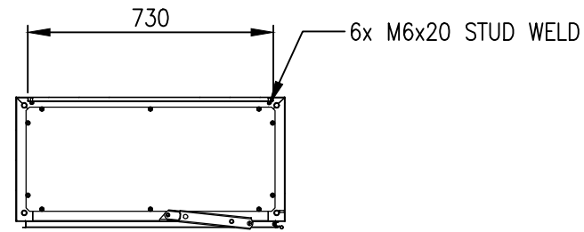
SECTION AV-AV
